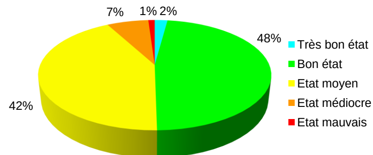
Figure 17 : Répartition des classes d'état pour l'IBD pour la période 2010-2011
