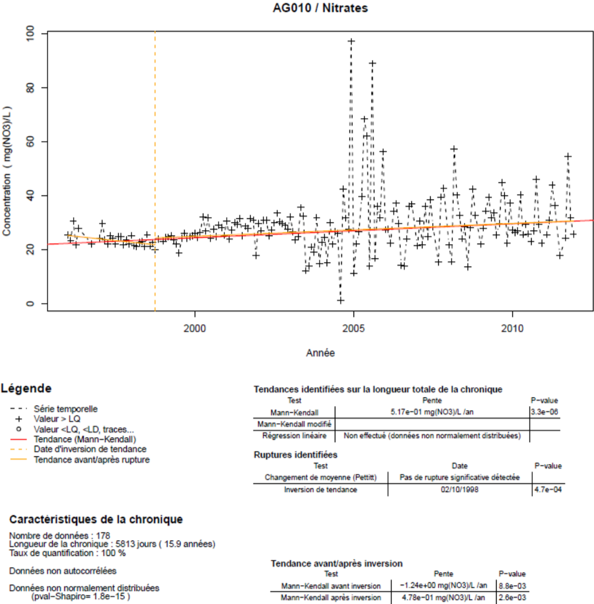
Figure 59 : Tendance à la hausse pour la craie du Cambrésis (FRARG010)
