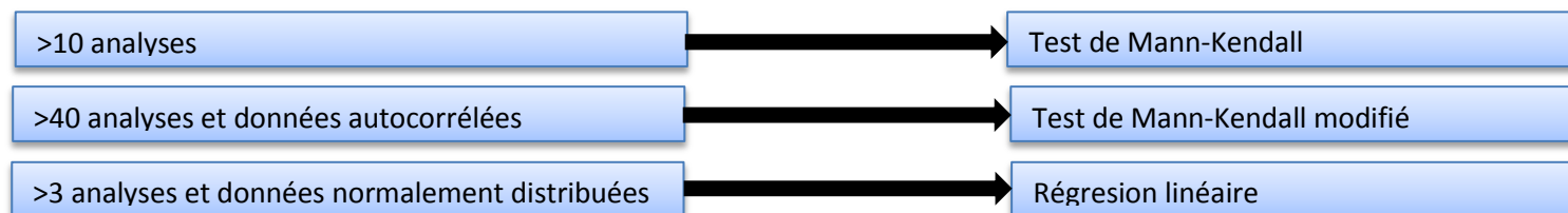
Figure 58 : Arbre décisionnel utilisé dans le module tendances de l'outil « HYPE ».
